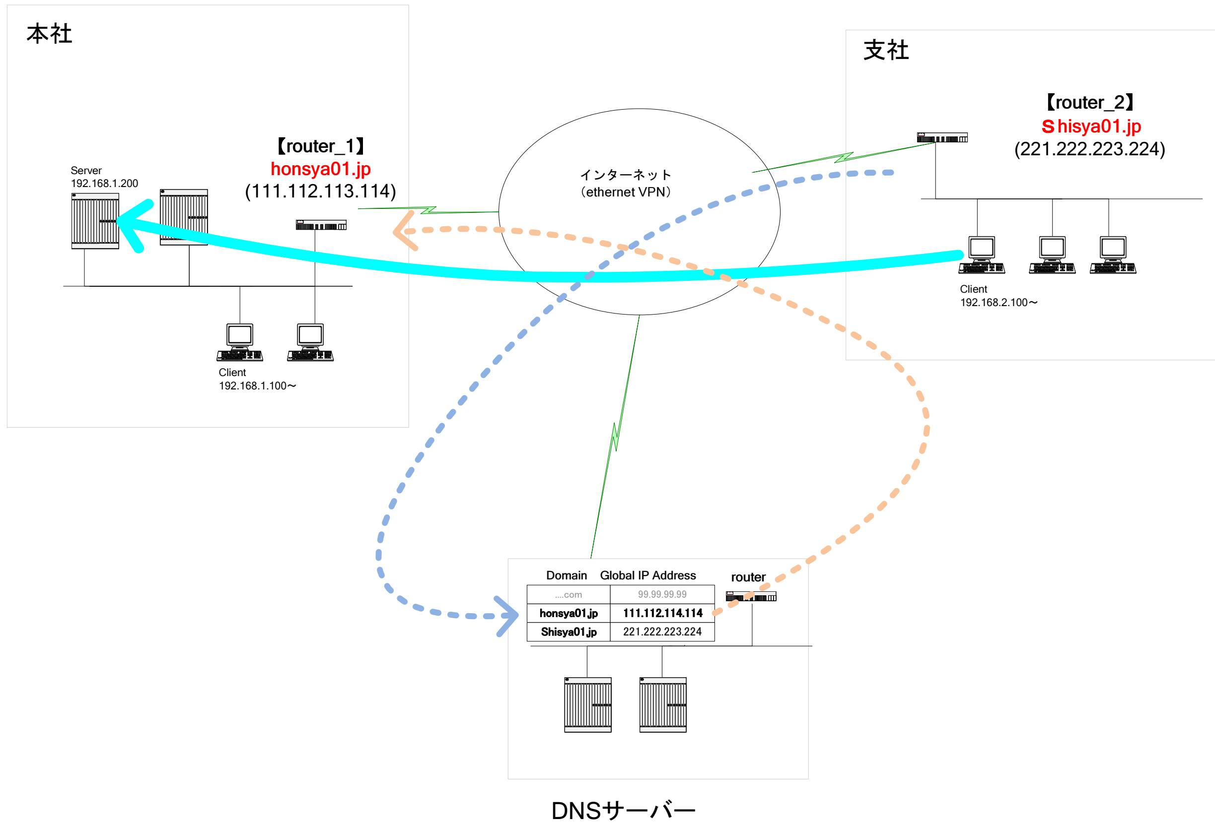
Ethernet VPN type2 (ルータにドメインを割り当てる)
